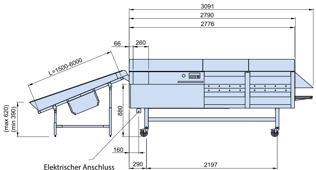
Pufferband seitlicher Anschluss
