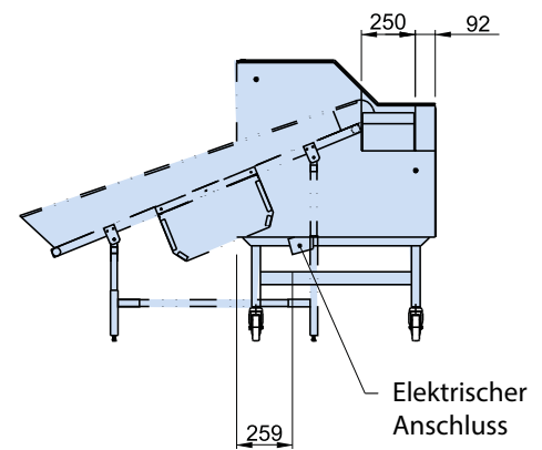
Pufferband Anschluss hinten
